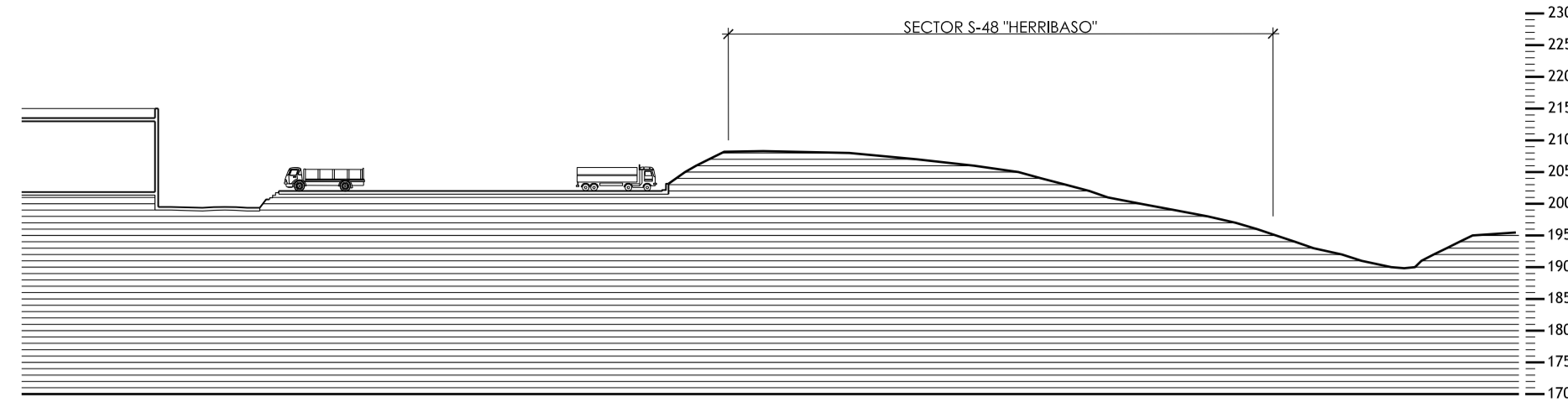
SECCIÓN TRANSVERSAL 1
