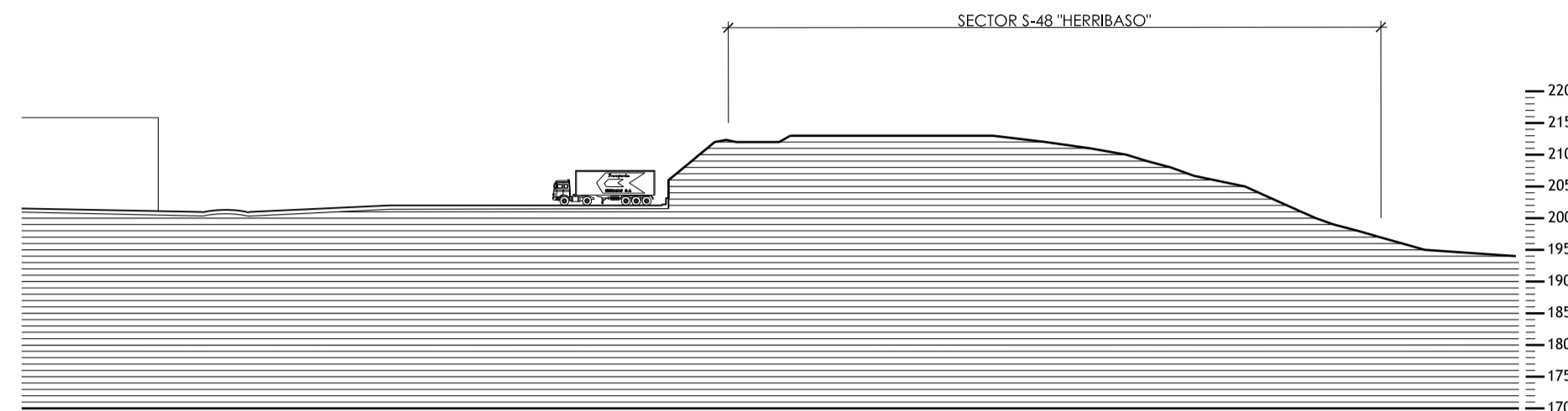
SECCIÓN TRANSVERSAL 2
